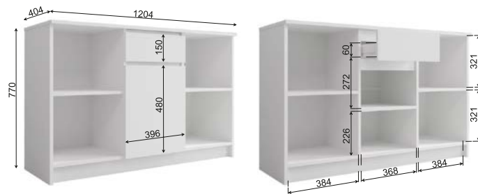
ТВ тумба «Мори» МТВ 1204.1
