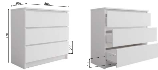
Комод «Мори» МК 800.1
