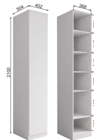
Модуль «Мори» MSH 400.1
