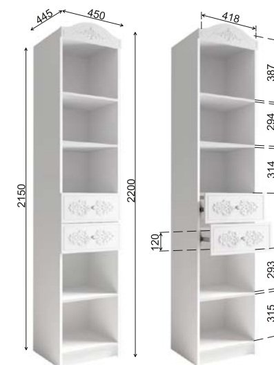
Модуль «Ki-Ki» СД 450.1
