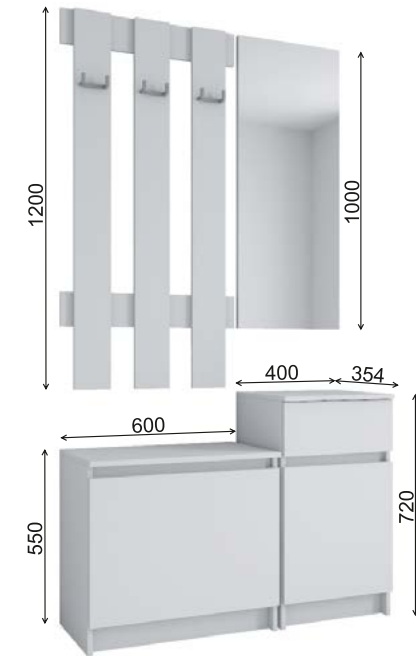
МС «Мори» общий вид
