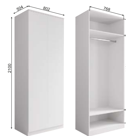
Модуль «Мори» MSH 800.1
