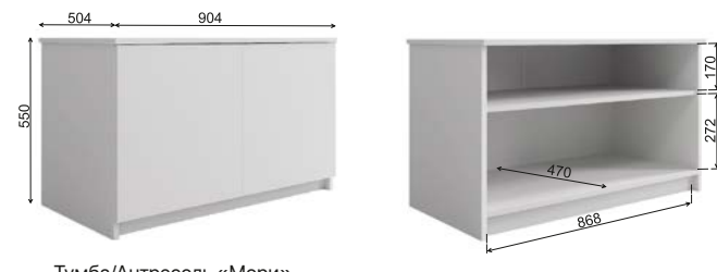
Тумба/Антресоль «Мори» МА 900.1
