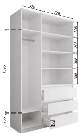
Модуль «Мори» MSH 960.1
