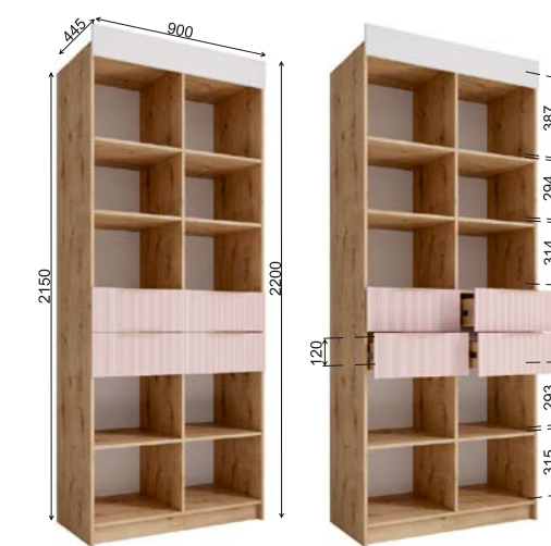
Модуль «Лавис» СД 900.1/2
