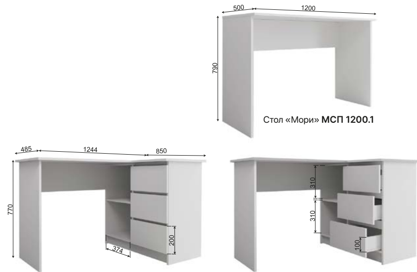
Стол «Мори» МС-16 универсальный
