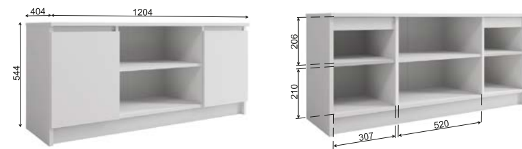
Модуль «Мори» МТВ 1200.1
