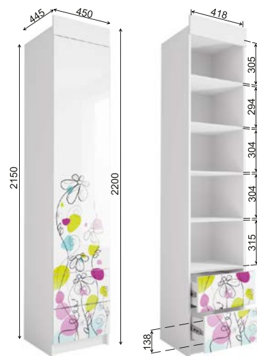
Модуль «Радуга» ШД 450.1
