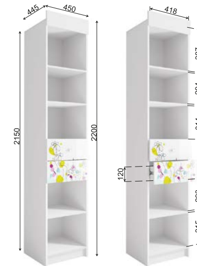
Модуль «Радуга» СД 450.1
