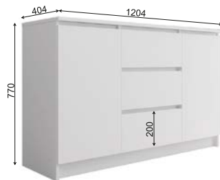
Модуль «Мори» MK 1200.3
