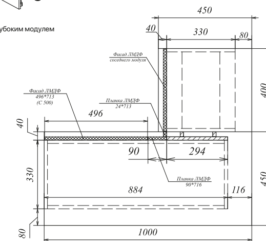
Стыковка столешниц модуля СУ 1050 с неглубокими модулями
