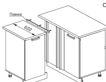
Стыковка столешниц модуля СУ 1000 с неглубокими модулями
