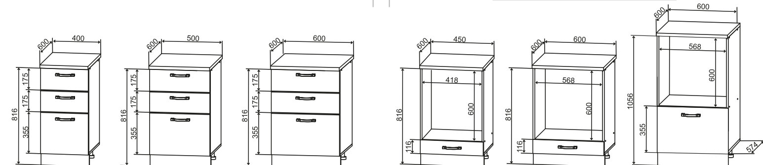
СЯШ 400 400/816/600 СЯШ 500 500/816/600 СЯШ 600 600/816/600 СДШ 450 450/816/600 СДШ 600 600/816/600 СН 600М 600/1056/600
