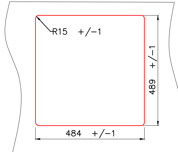
Врезной монтаж мойки (I)
